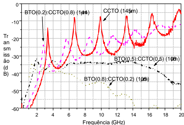
Figura 2 - Espectro de transmissão dos ressonadores CPW medidos com os diversos filmes.
