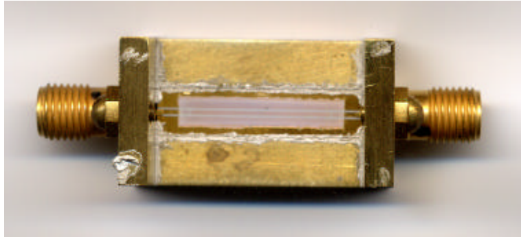
Figura 1 - Circuito ressonador linear CPW montado com filme dielétrico depositado.
