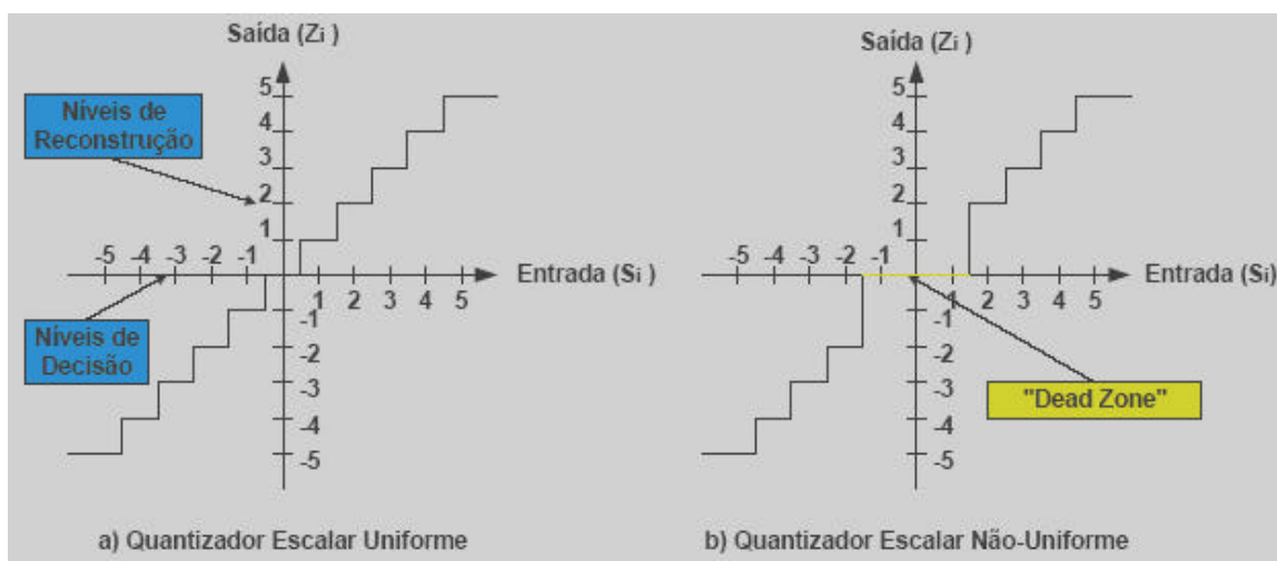
Figura 2.6: Quantizadores escalares. [5]
